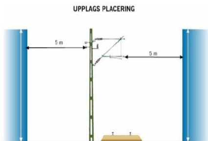
Figur 2. Exempel på tillåten placering av upplag vid elektrifierade spår.
